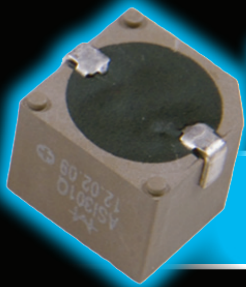
SMT Buzzer
